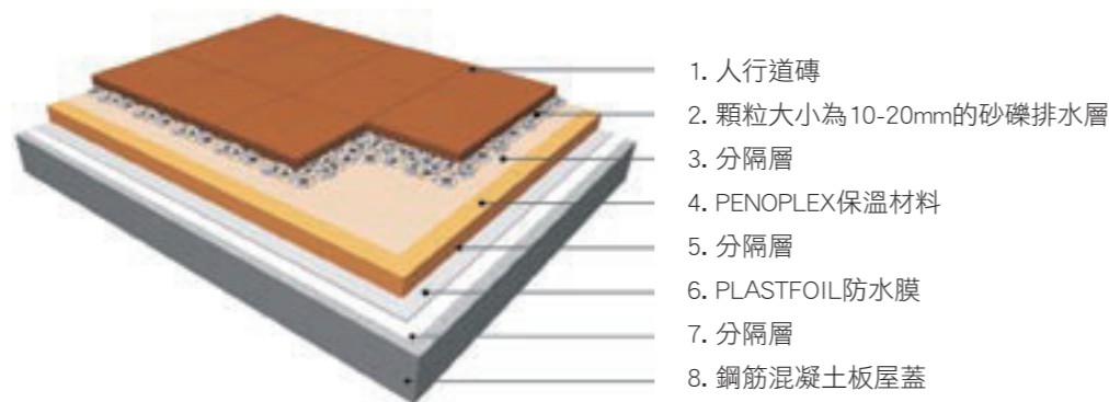
（圖四）鋪人行道磚的倒置式上人屋面
