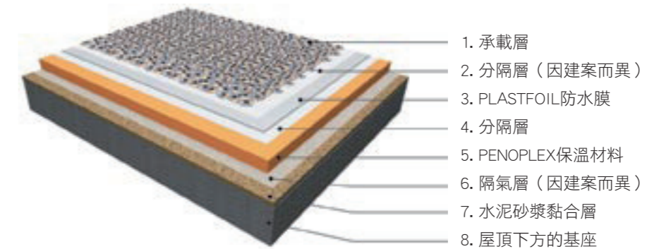
（圖二）壓頂屋面的防水層
