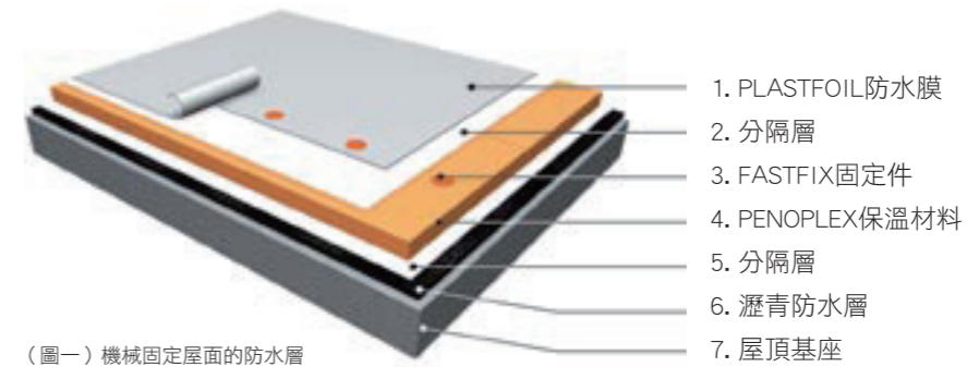
（圖一）機械固定屋面的防水層
